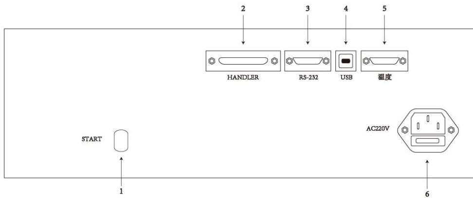
图3-4 后面板
