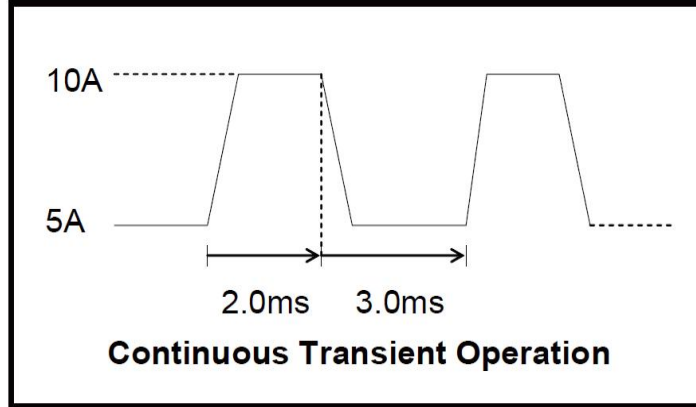
A值10A、A脉宽时间2.0mS、B值5A、B脉宽时间3.0mS
